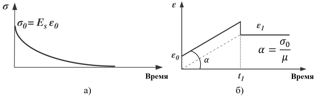
Рисунок 6 – Графические зависимости модели Максвелла: а) релаксация, б) ползучесть, t_1 – момент времени, в который снимается нагрузка
